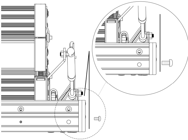
FIGURA 5 : INSTALACIÓN DE CORREA METÁLICA
