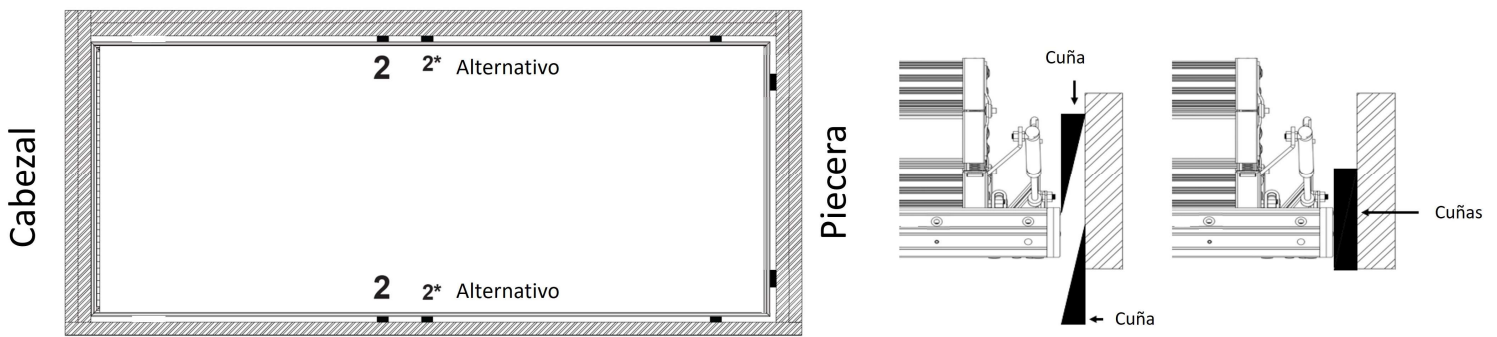
FIGURA 25 : COLOCACIÓN DE CUÑAS EN MARCO LATERAL
