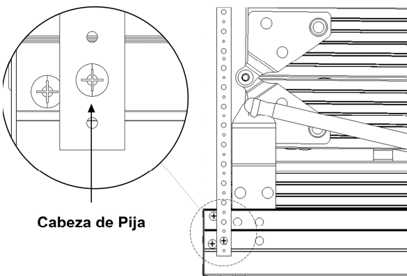
FIGURA 6: POSICIÓN DE LA CORREA METÁLICA
