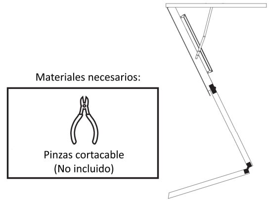
FIGURA 27 : DESPLIEGUE DE SECCIONES DE ESCALERA
