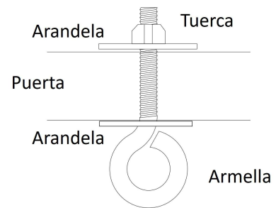
FIGURA 21 : ASEGURANDO ARMELLA
