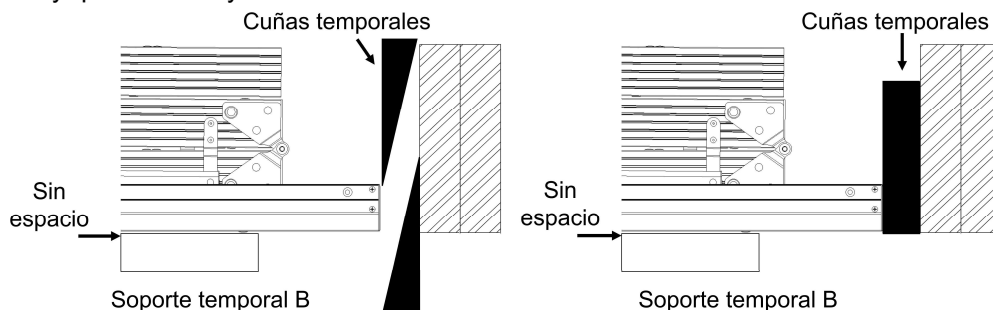
FIGURA 12 : COLOCACIÓN DE CUÑAS EN LA PIECERA
