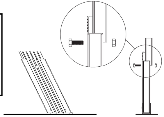
FIGURA 29 INSTALACIÓN DE TACÓN DE ALUMINIO
