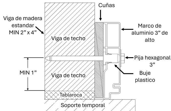
FIGURA 2 REQUISITOS DE VIGA DE TECHO
